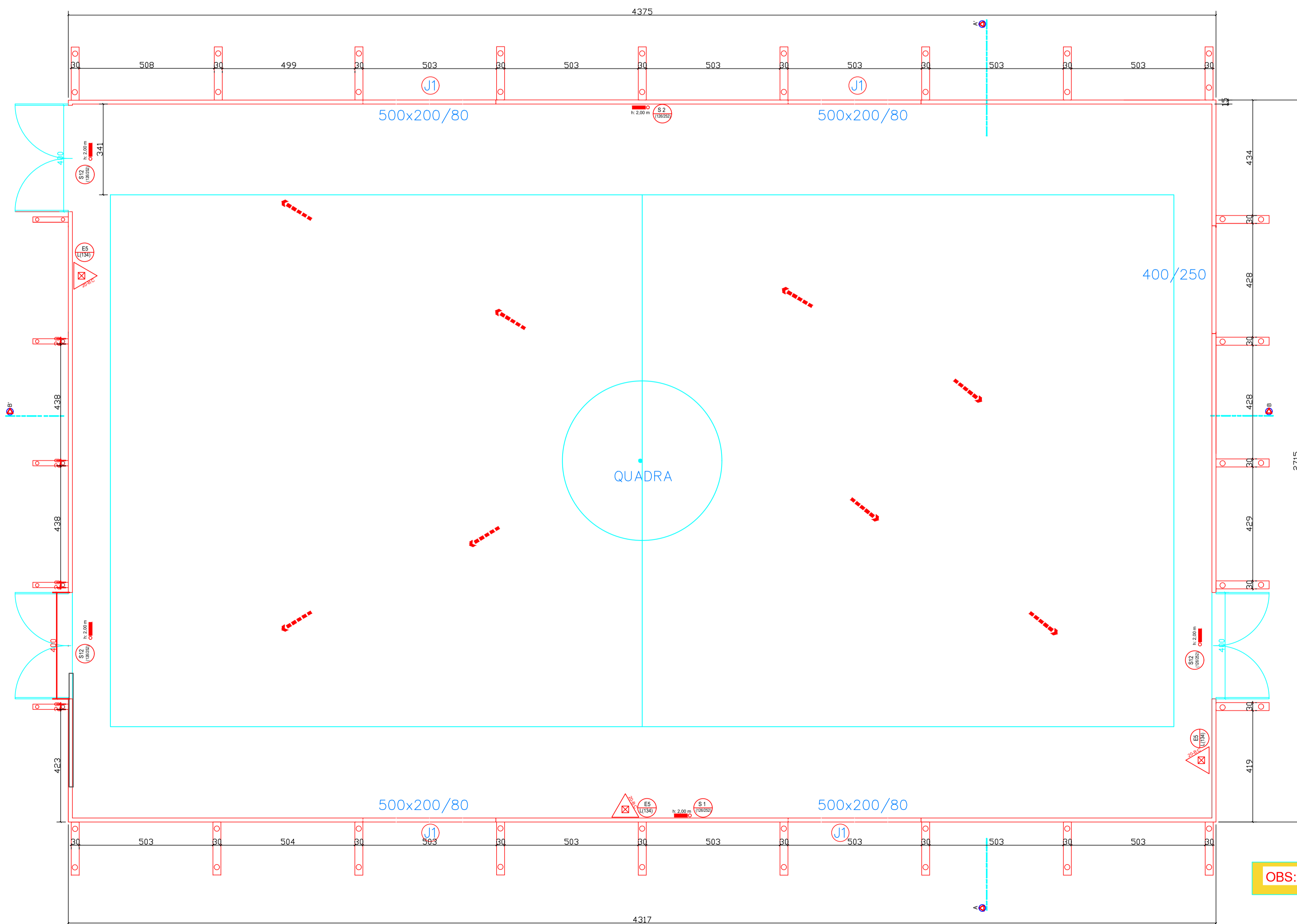
PLANTA BAIXA ESCALA: 1:100
