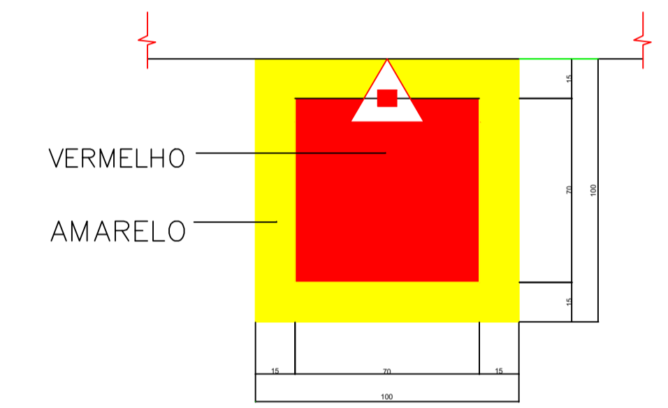
DETALHE PISO
