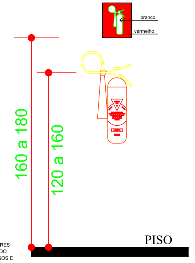
DETALHE EXTINTOR ESCALA: 1:20
